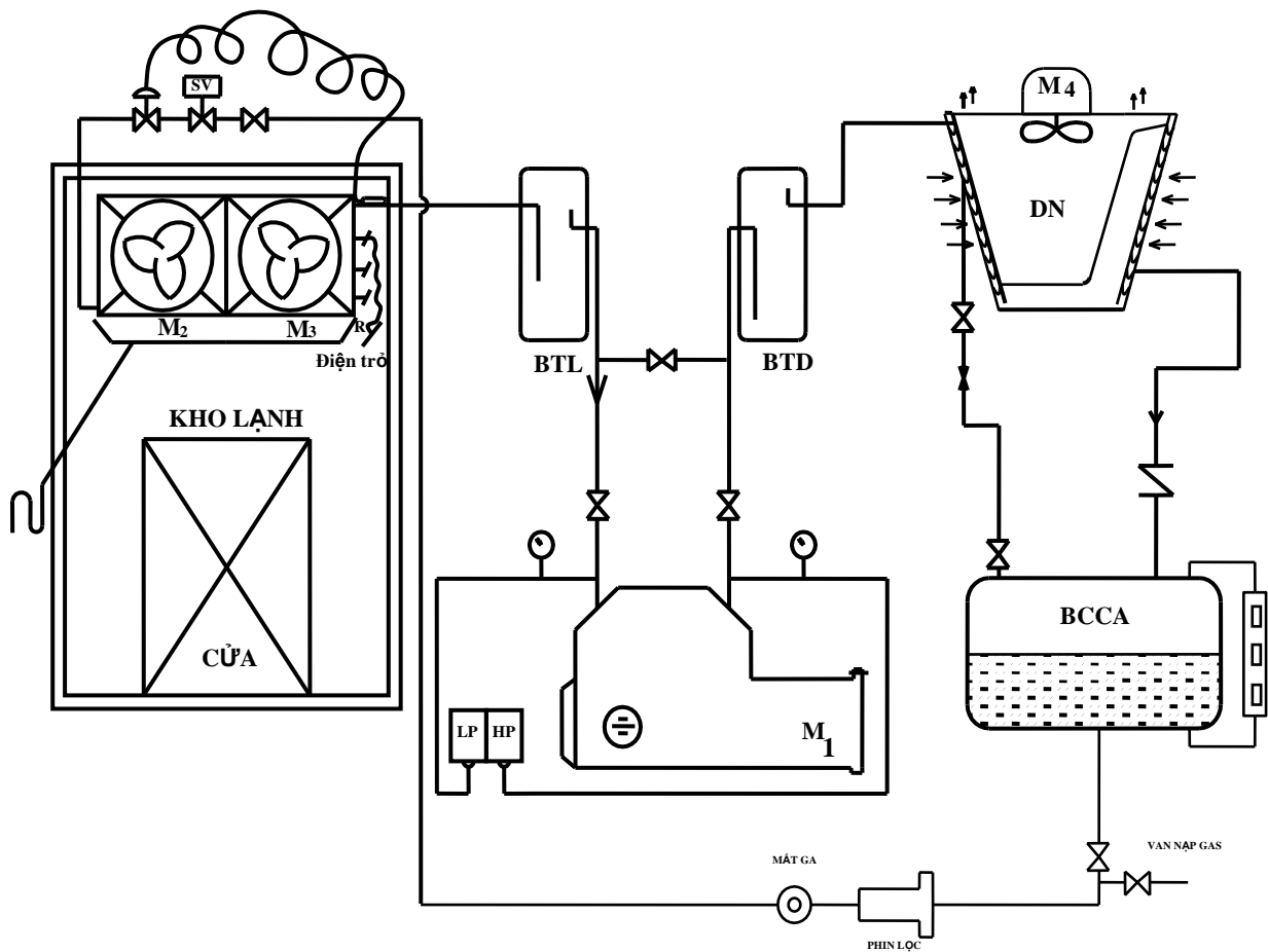
SƠ ĐỒ HTL/ KHO LẠNH
