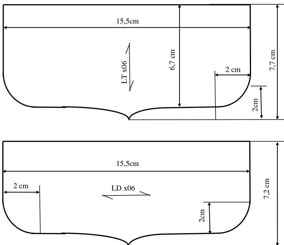
Hình 2. Bản vẽ các chi tiết bán thành phẩm
